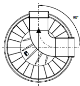
Bodem met stroomprofiel 90°
